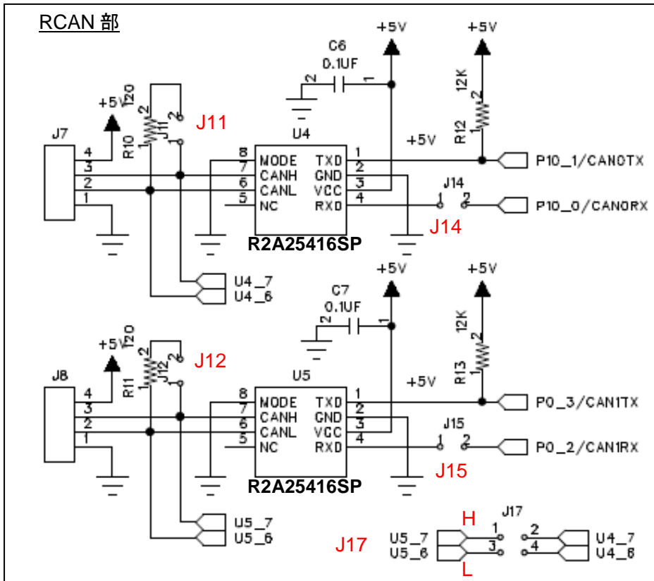
図 2-3 RCAN インタフェース部(回路図)
