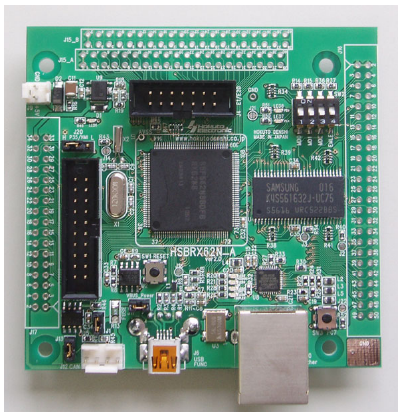
写真は HSBXR62N-A シリーズです。HSBRX621-A シリーズには Ethernet 及び関連の部品は未実装となります
