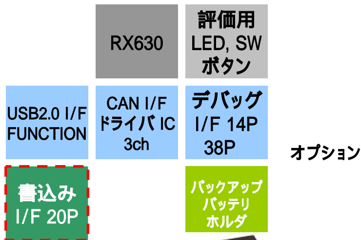
<144ピンMCU搭載ボードブロック図>
