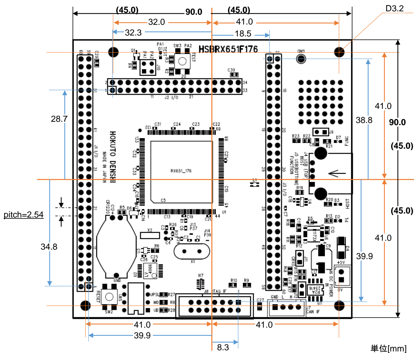
図 3-1 ボード寸法図
