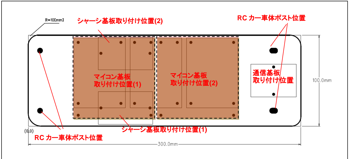
図 1-1(a) ボード配置図
