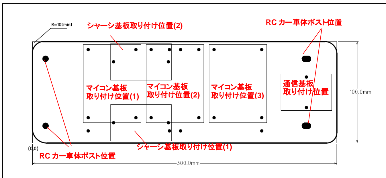
図 1-1 ボード配置図
