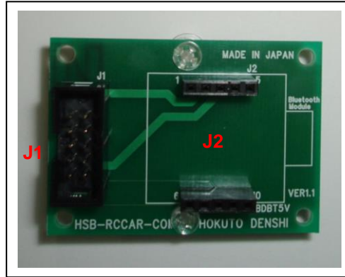
図 1-7 ボード配置図
