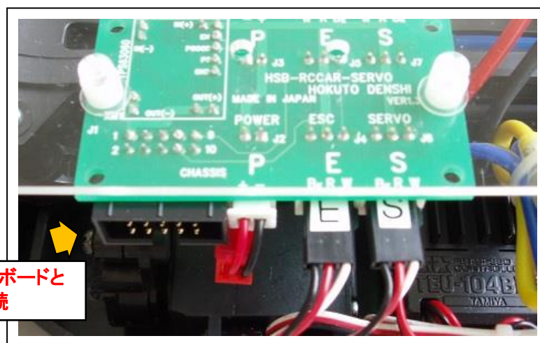
図 1-5 シャーシ基板ケーブル接続イメージ(改造後)
