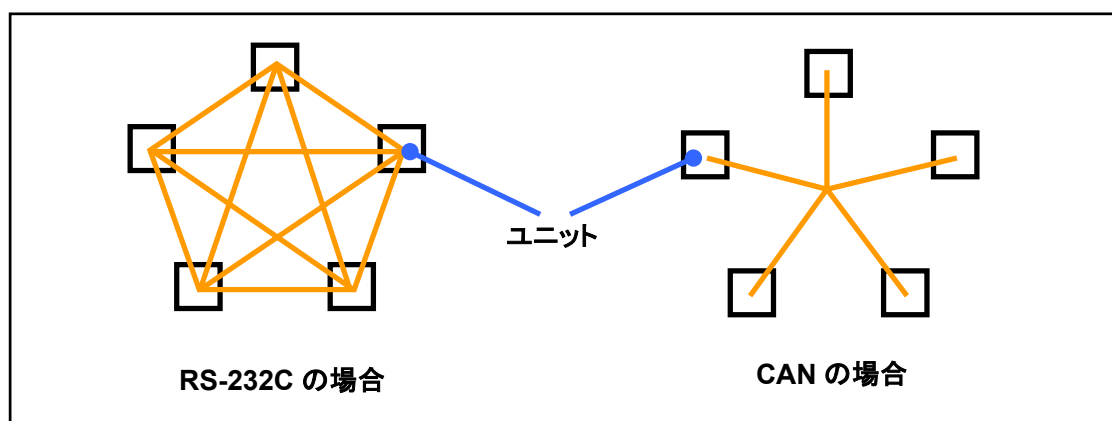
図 2-1 RS232C と CAN のネットワーク接続の比較
