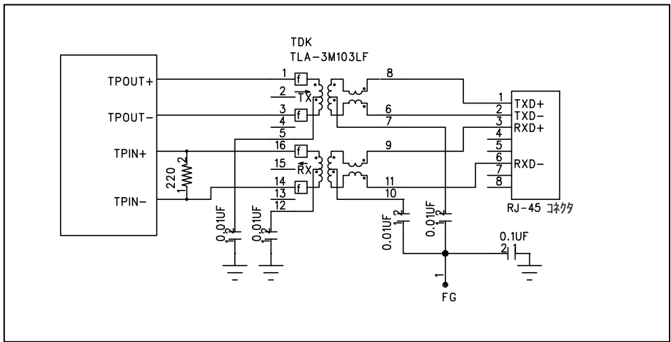
図 2.19 RTL8019ASと RJ-45 コネクタの接続
