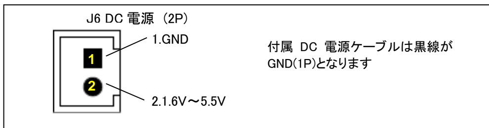
図 4-2 DC 電源図
