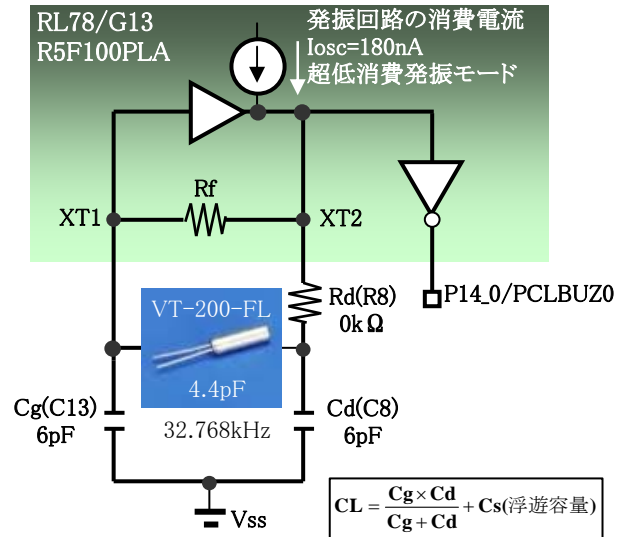
図2.評価回路図
