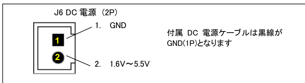
図 2-2 DC 電源図
