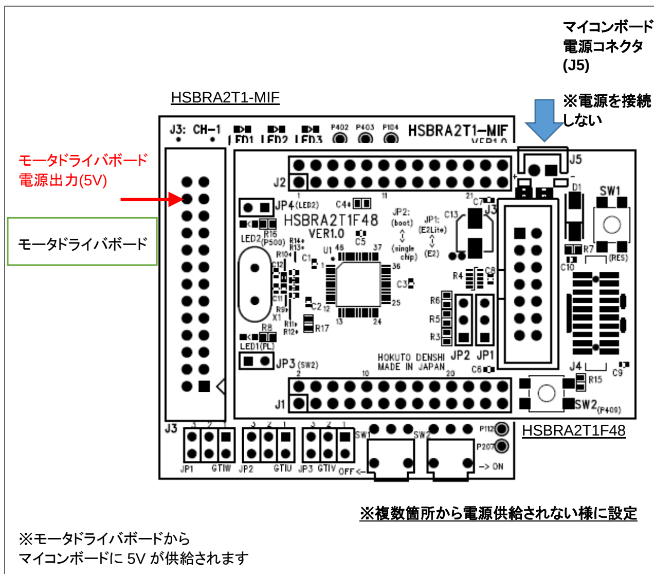
図 電源供給方法イメージ図
