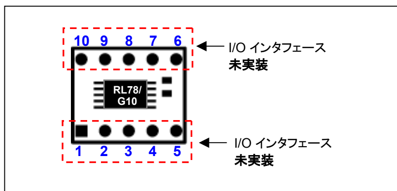
図 4-1 ボード配置図
