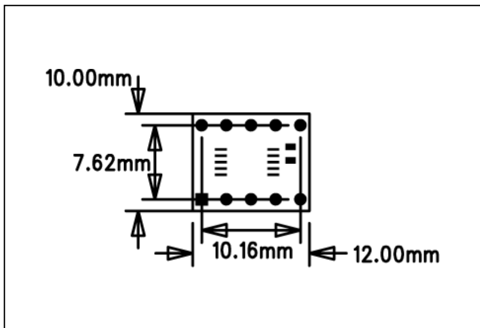
図 7-1 寸法図
