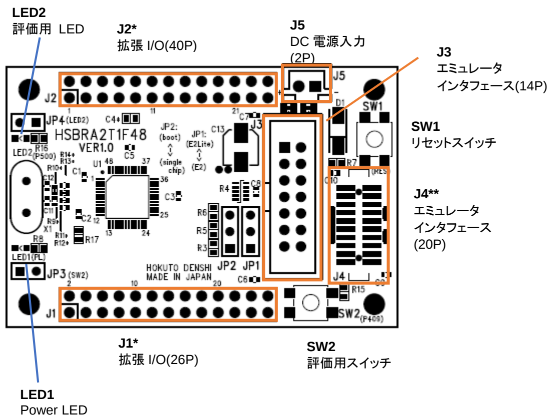
図 1-1 ボード配置図
