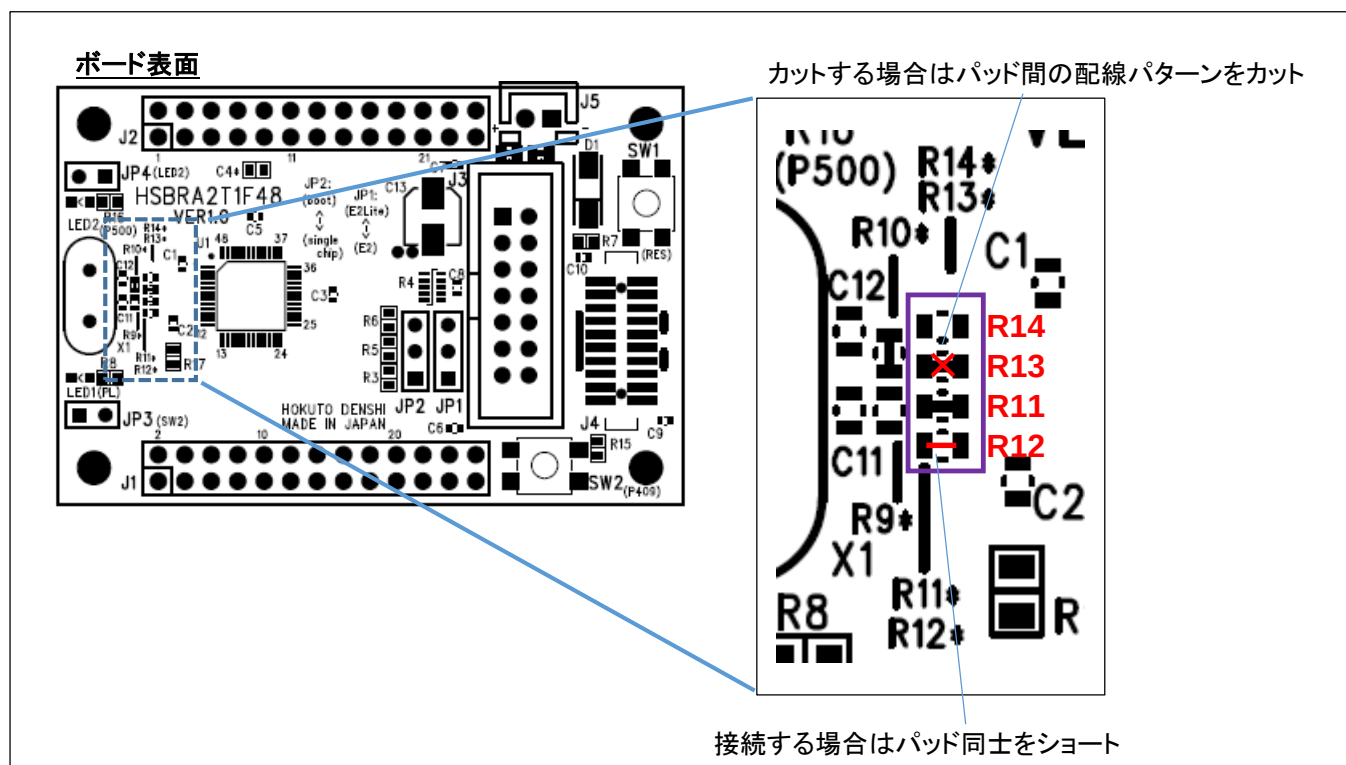
図 2-5 P212, P213 接続
