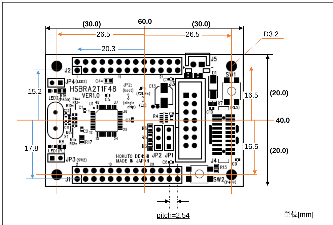
図 3-1 ボード寸法図
