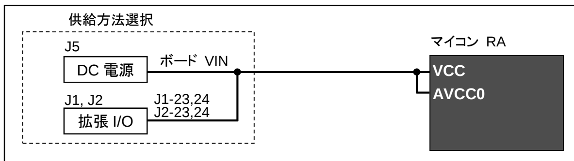
図 2-2 電源供給方法イメージ図
