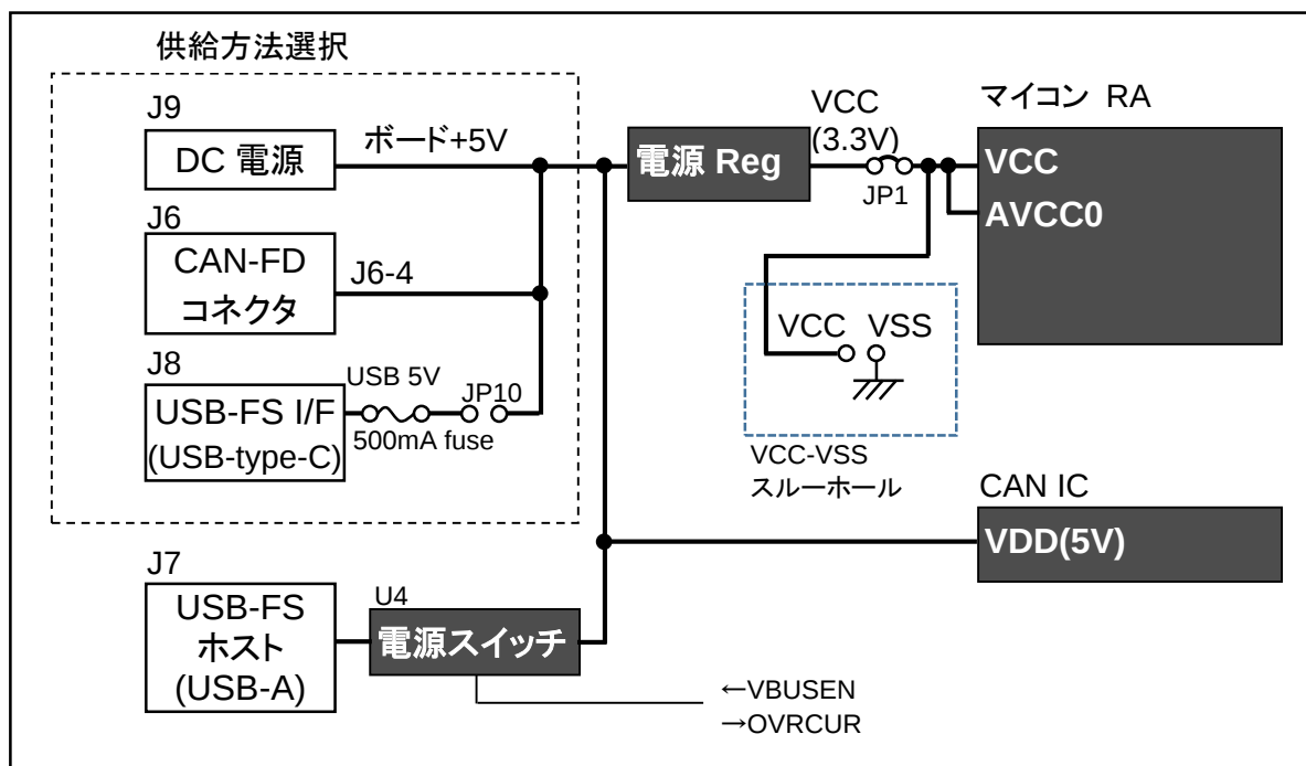
図 2-2 電源供給方法イメージ図
