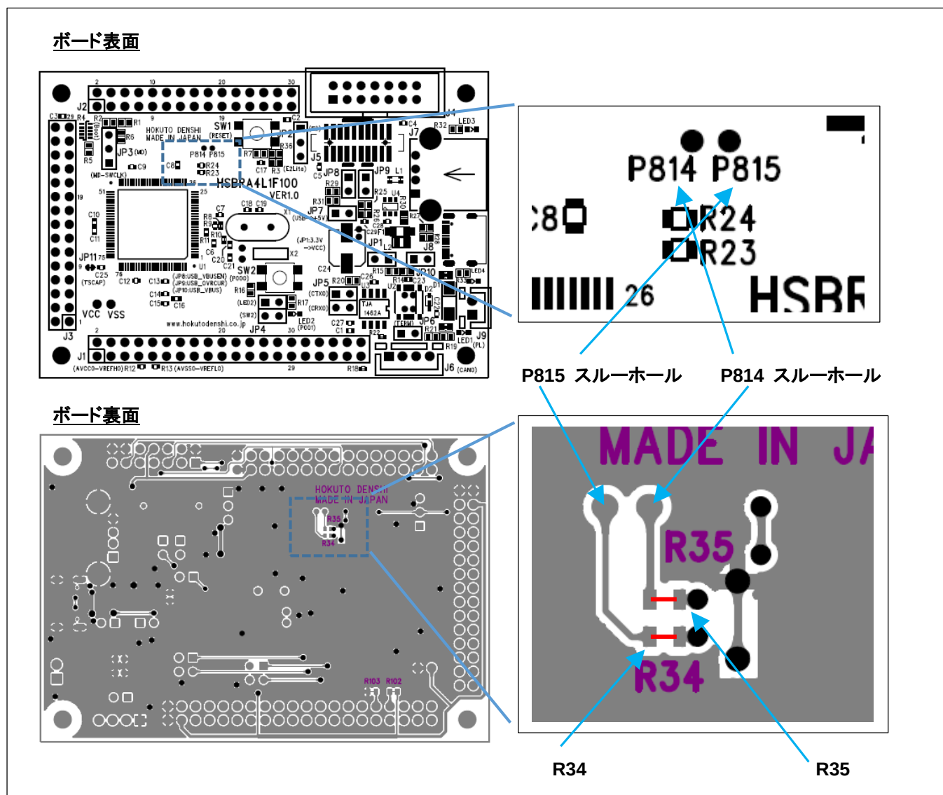
図 2-5 USB_DP/DM, P814, P815 接続
