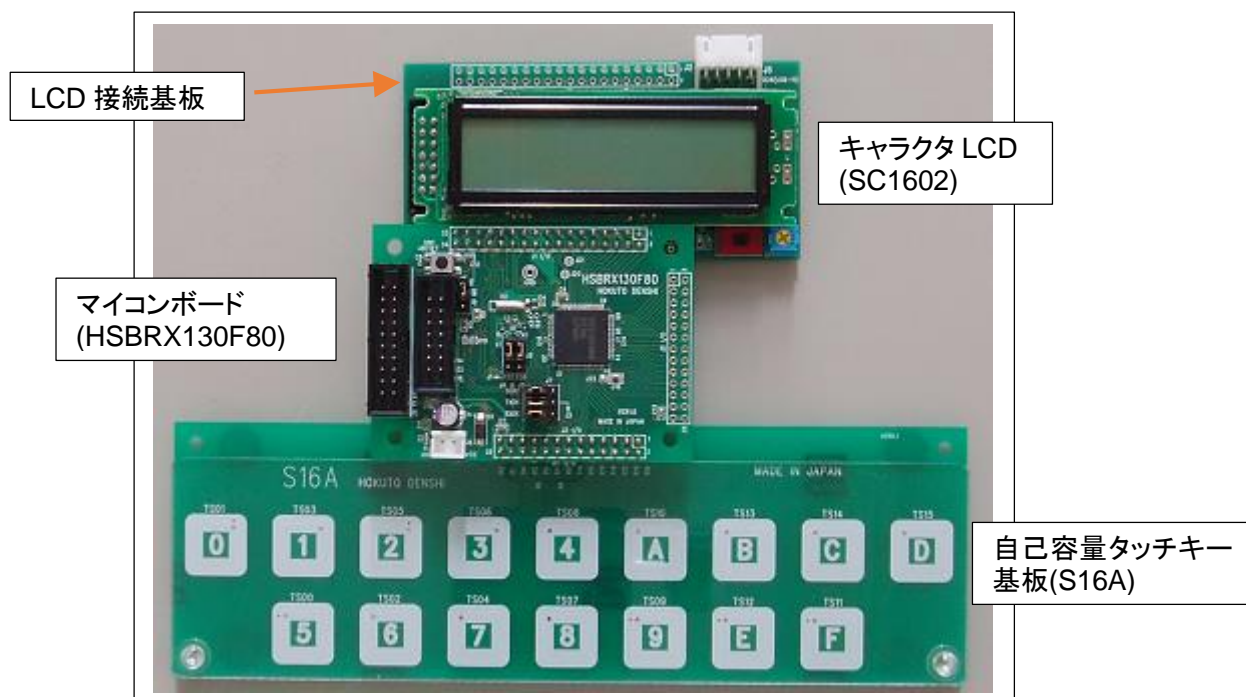
図 2-1 接続例(S16A)
