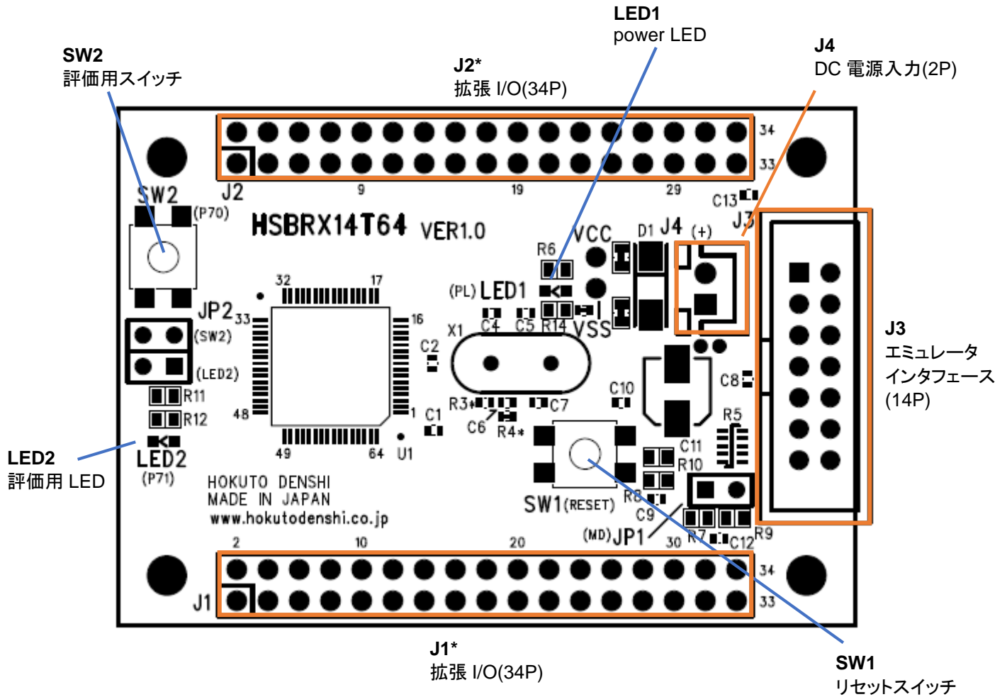
図 1-1 ボード配置図
