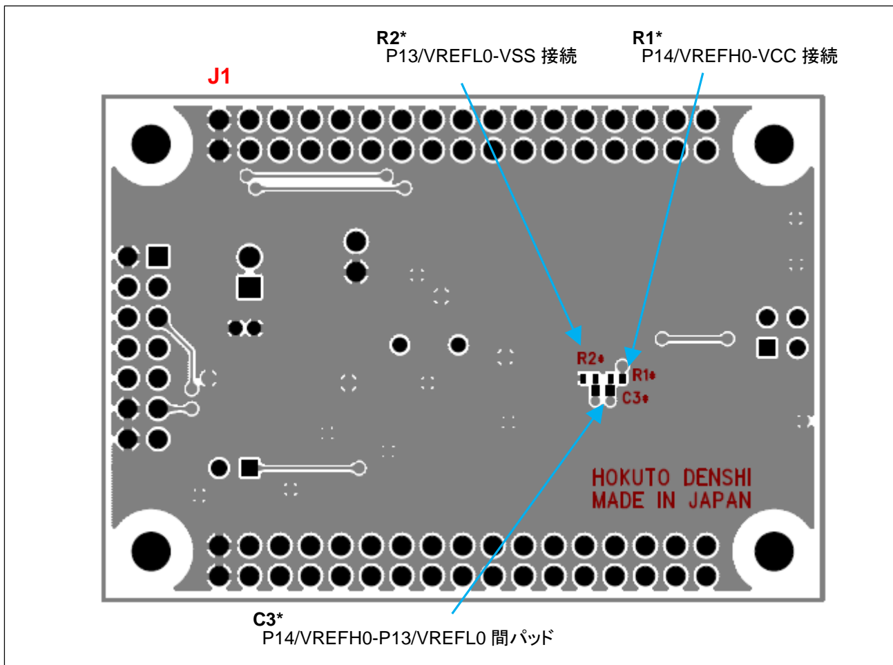
図 2-4 基板裏面の C3, R1, R2 部
