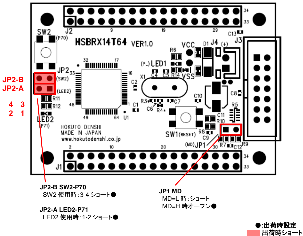
図 1-2 ボード配置図(ジャンパ)
