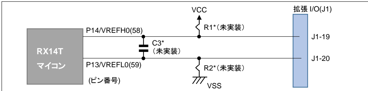
図 2-3 VREFH0, VREFL0 接続
