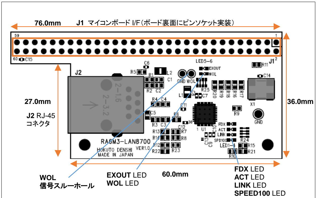
図 1-2 ボード外形(RA6M3-LAN8700)
