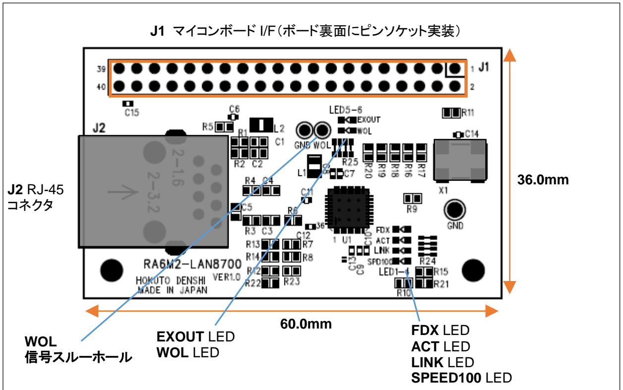
図 1-1 ボード外形(RA6M2-LAN8700)
